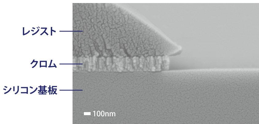
エッチング処理後の断面SEM像
