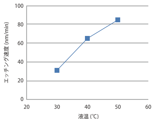
クロムエッチング速度
